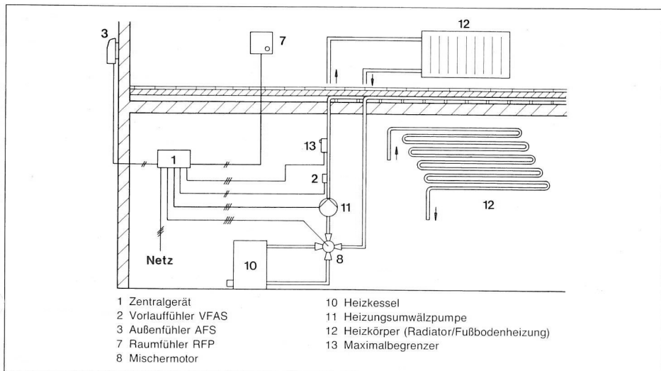
3 Anlagenschema — Mischbetrieb
