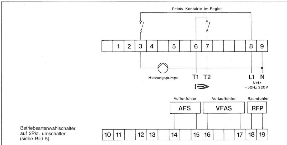
9 Elektrischer Anschlußplan — Brennerbetrieb
