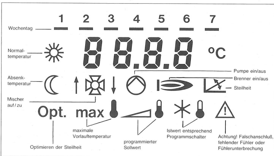
14 Anzeige mit allen möglichen Symbolen und Erläuterungen
