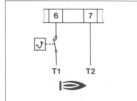
11 Anschluß des Maximalbegrenzers — Brennerbetrieb
