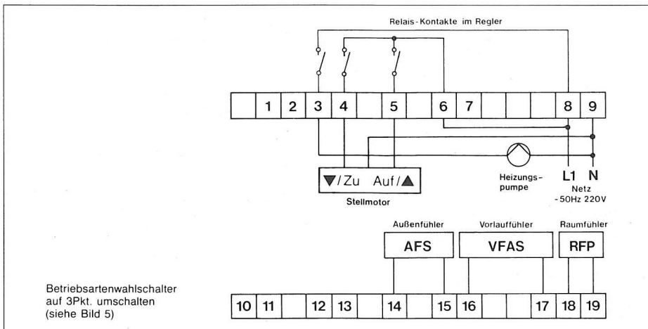
10 Elektrischer Anschlußplan — Mischerbetrieb
