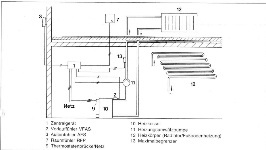
2 Anlagenschema — Brennerbetrieb
