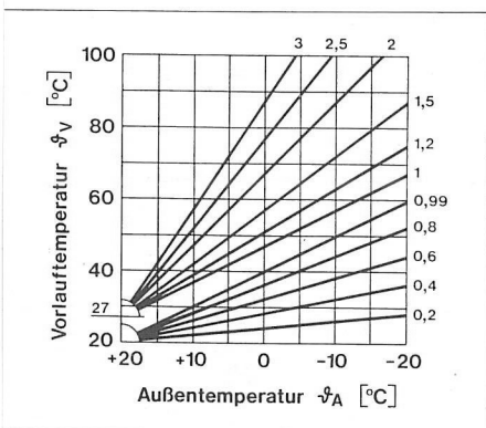
13 Heizkurven
