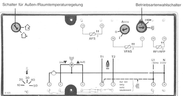
5 Regleroberteil — Rückseite
