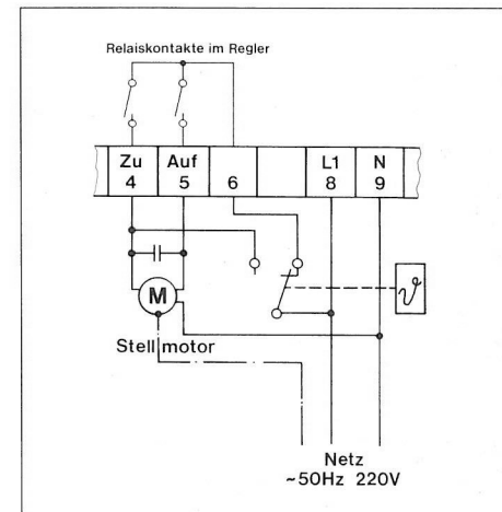
11a Anschluß des Maximalbegrenzers — Mischerbetrieb
