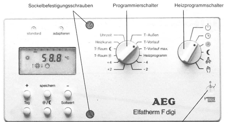
Schalter für Aufheizoptimierung
