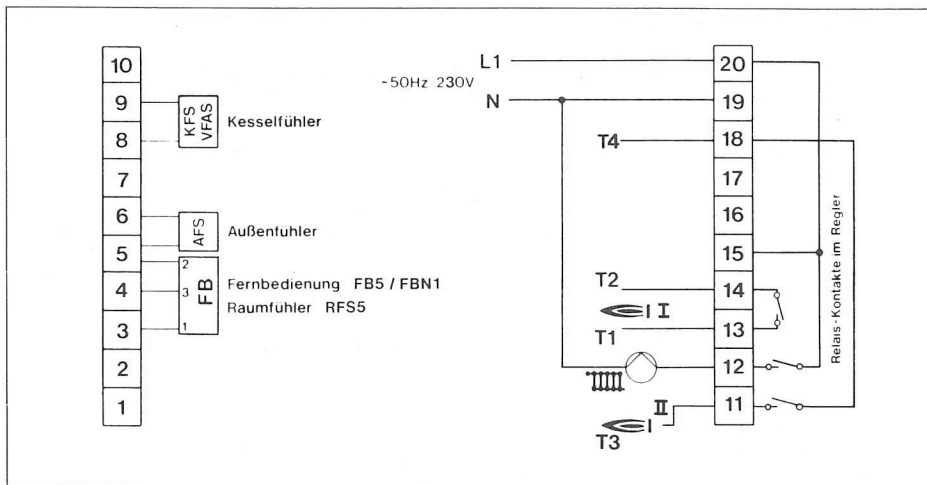
10 Anschlußschema Elfatherm E22ZKP
