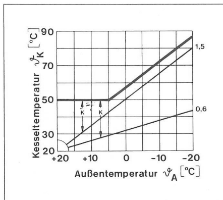
20 Diagramm „Minimalbegrenzung“
