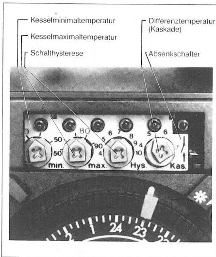
14 Frontansicht — Einstellregler und Schalter
