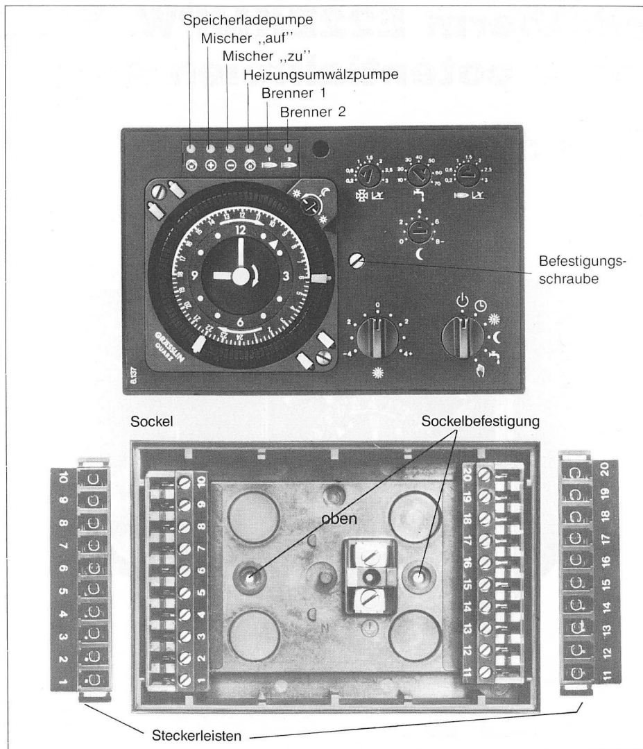
3 Frontansicht mit separatem Sockel bzw. Steckerleisten
