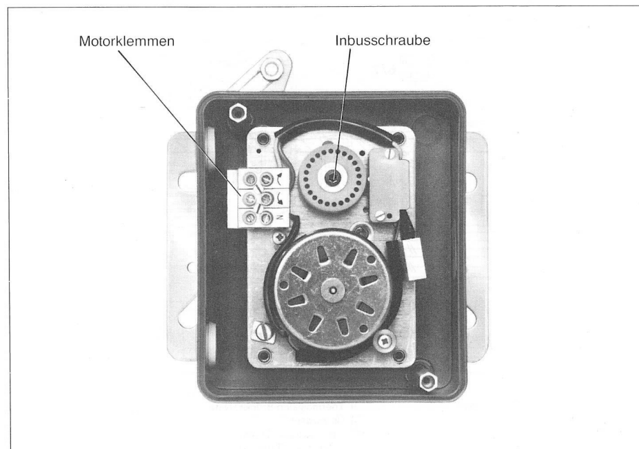
4 Stellmotor SM75
