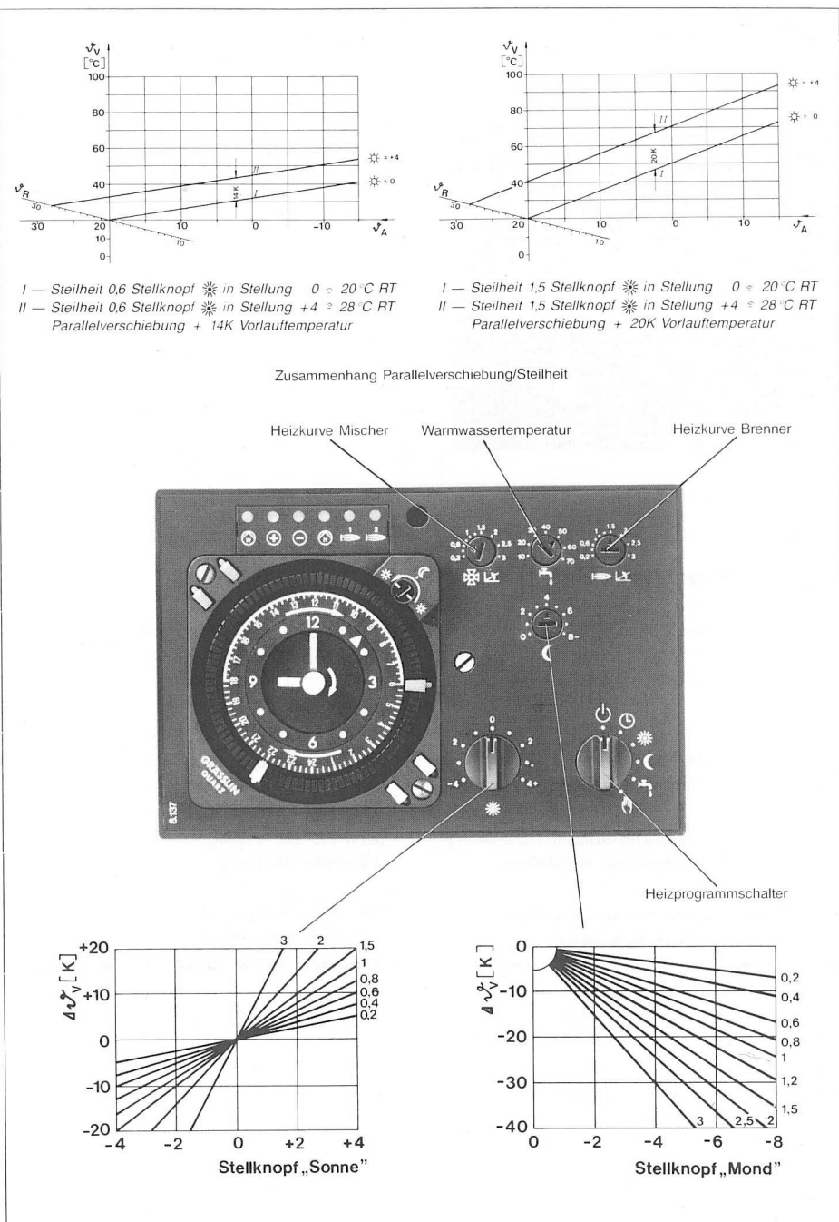
17 Reglerfrontansicht — Einstellknöpfe
