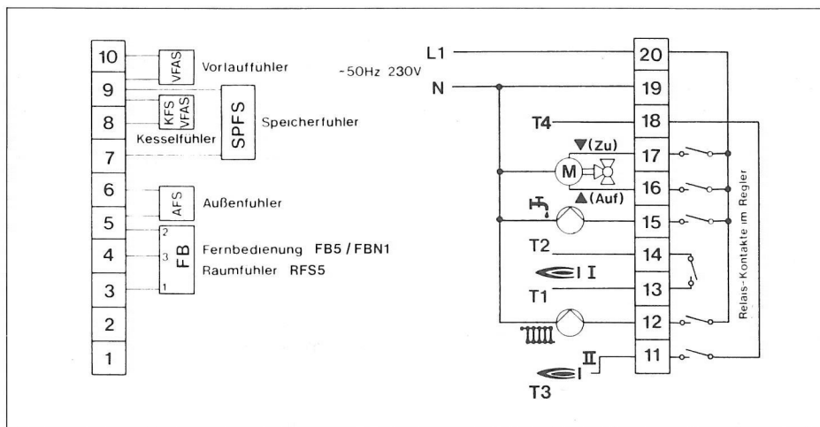
11 Anschlußschema Elfatherm E22ZKMPW
