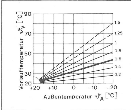
19 Heizkurve Flächenheizung
