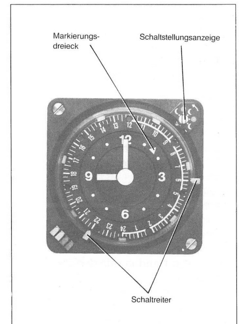
22 Quarzschaltuhr/Tagesprogramm mit Gangreserve
