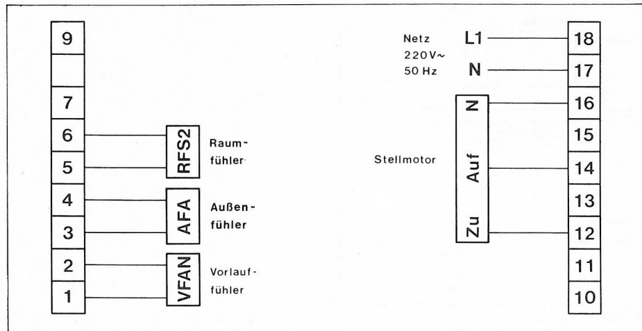
Bild 6 Anschlußschema zu 2.2.1
