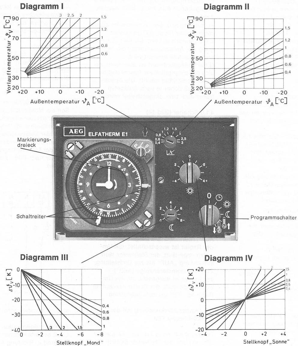
Bild 14 ELFATHERM E1M — Frontansicht mit Diagrammen
