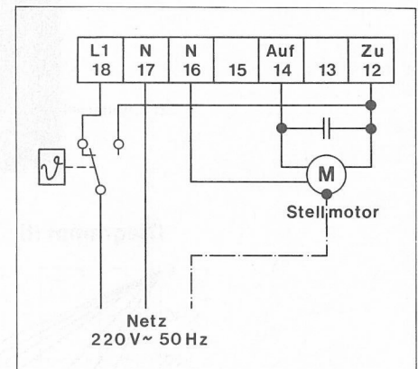
Bild 13 Anschlußschema Maximalbegrenzer
