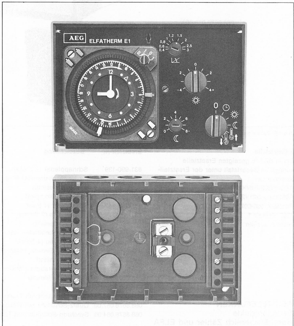
Bild 11 Zentralgerät E1M mit Grundplatte
