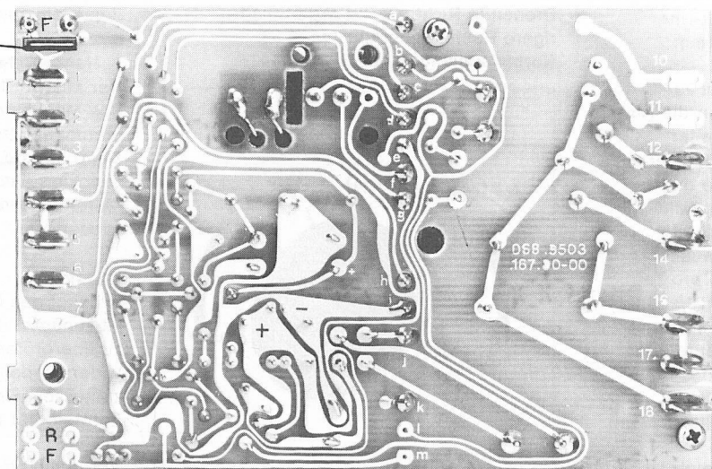
Bild 15 ELFATHERM E1M — Ansicht auf Leiterplatte
