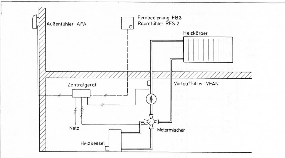
Bild 2 Anlagenschema ELFATHERM E1M — Radiatorenheizung
