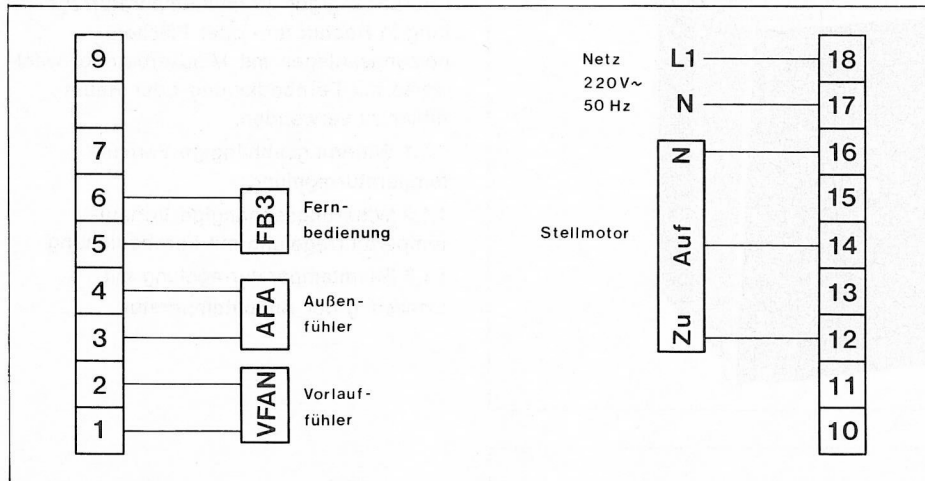
Bild 5 Anschlußschema zu 2.1.2
