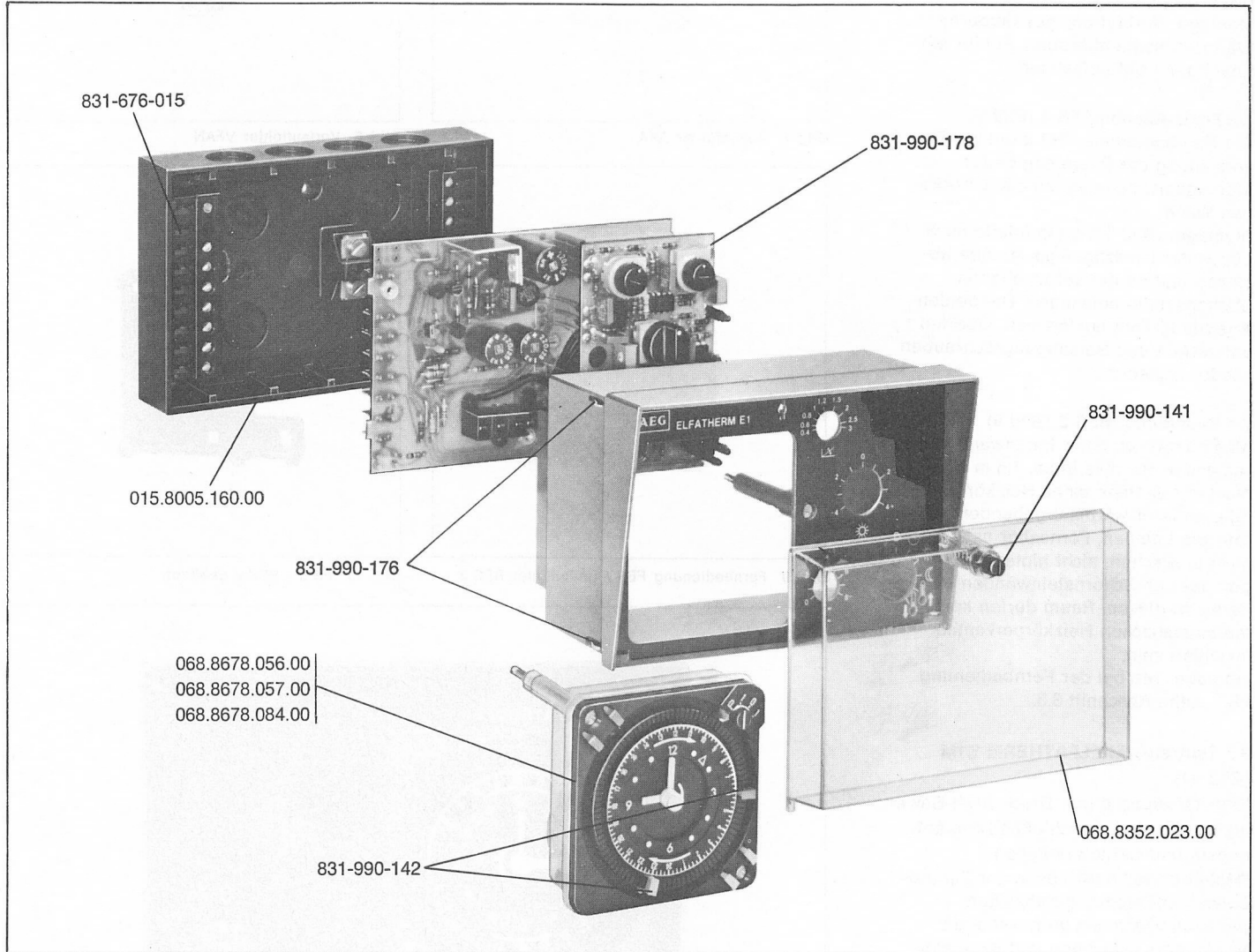
Bild 16 Zentralgerät ELFATHERM E1M, Ersatzteile
