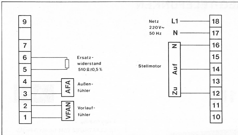
Bild 4 Anschlußschema zu 2.1.1
