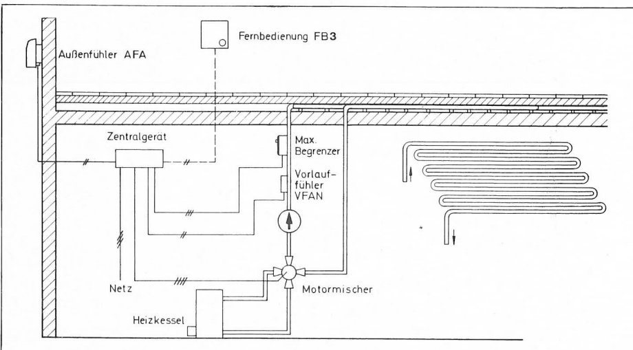
Bild 3 Anlagenschema ELFATHERM E1M — Fußbodenheizung
